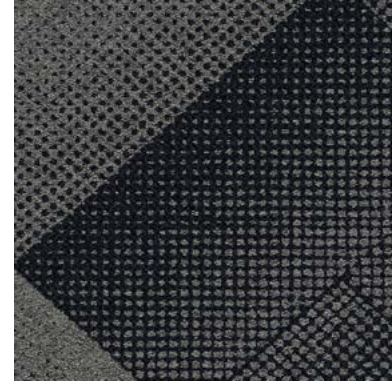
107185 Carbon
