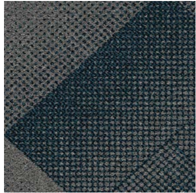
107184 Cobalt
