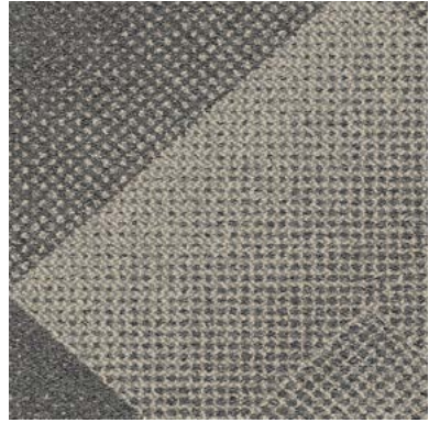
107181 Oxygen
