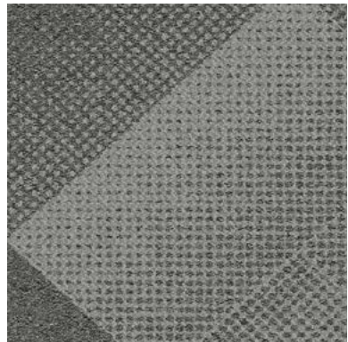
107183 Titanium
