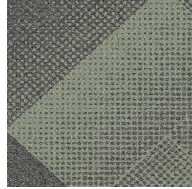
107182 Beryllium
