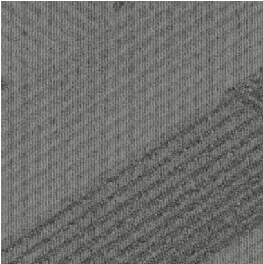
107178 Selenium
