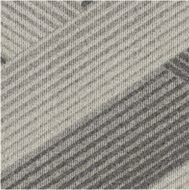
107176 Zinc
