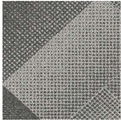
107180 Xenon
